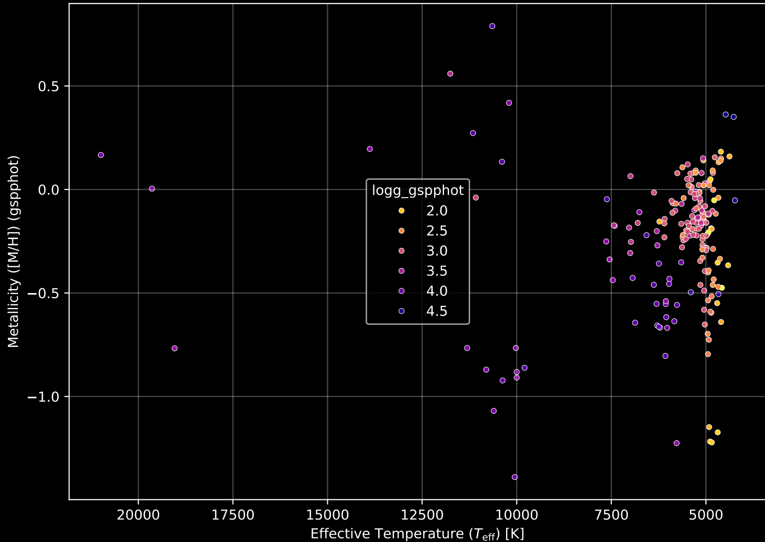
APOGEE DR17 Field: [M35N2158] Stellar Population Parameters (n= 201)
